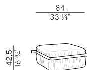
925/O80-OUT pouf \ pouf
