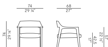
906/PLI poltrona lounge \ lounge armchair
