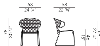
698/P \times 6 poltroncina impilabile \ stackable armchair
