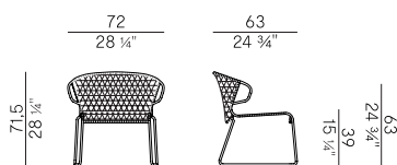
698/LP \times 4 poltrona impilabile \ stackable lounge chair
