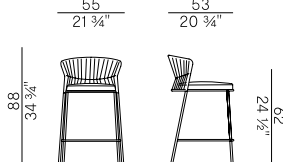
923/S sgabello basso impilabile \ stackable counter stool
