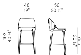
942/AW sgabello alto \ barstool
