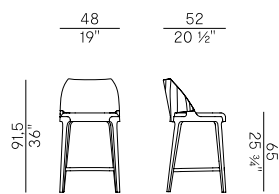
942/SW sgabello basso \ counter stool
