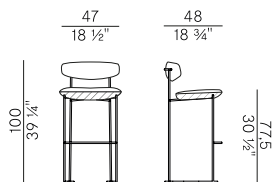
922/AMB-OUT sgabello alto \ barstool
