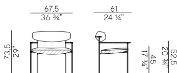
922/LMB poltrona lounge \ lounge armchair
