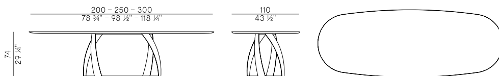
770/TG-O tavolo \ table
