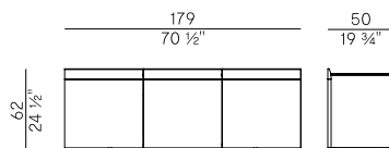
884/MB2-180 madia \ sideboard
